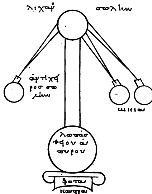
FIGURE 15. — Alambic à trois récepteurs. Réduction aux 2/3.
